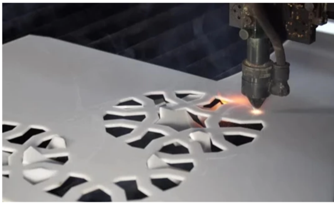
CO2 laser cutting
